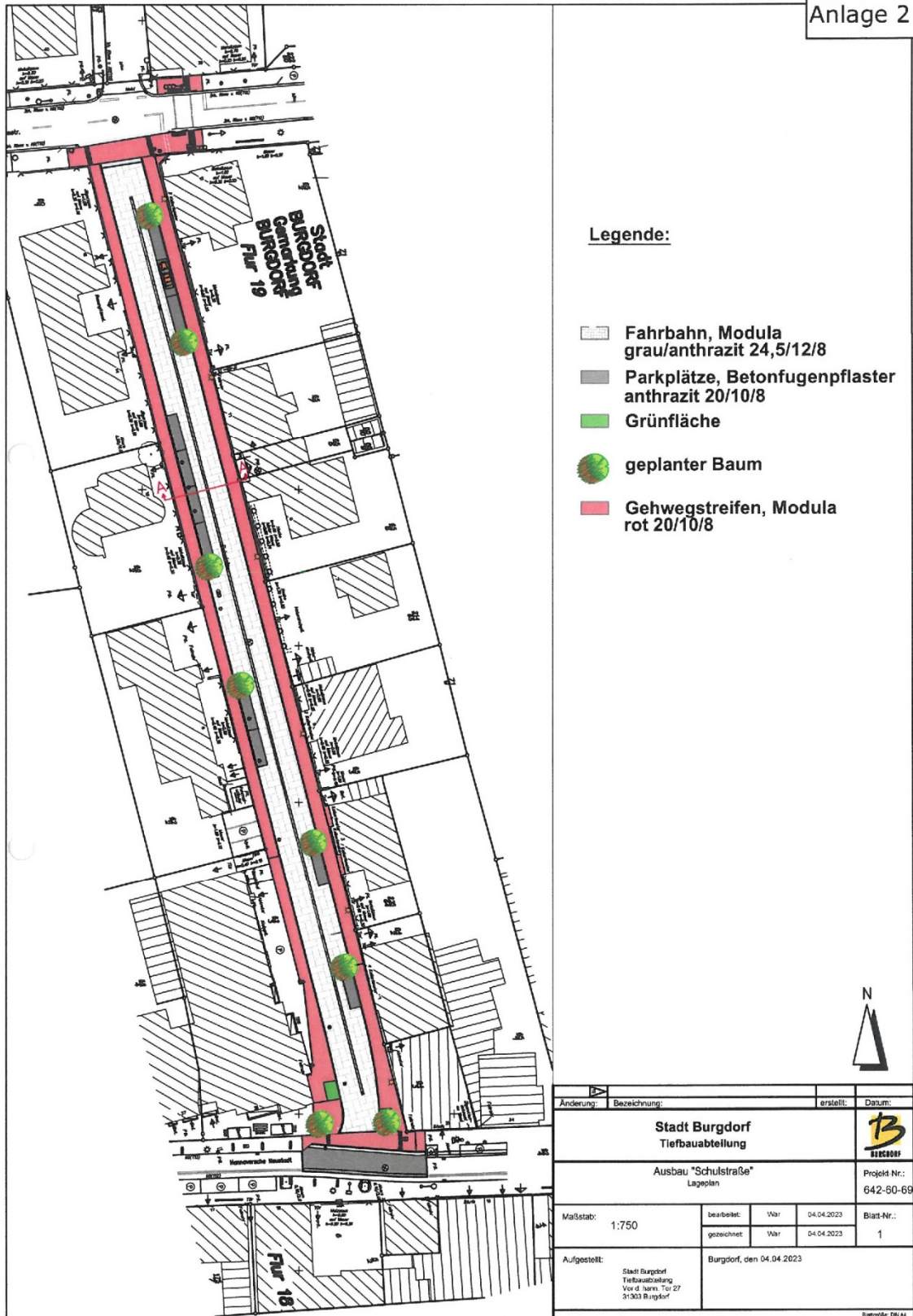
Abbildung: Ausbauplanung der Schulstraße (Anlage aus BV 2023 0468) – Lageplan. Darstellung: Stadt Burgdorf.
